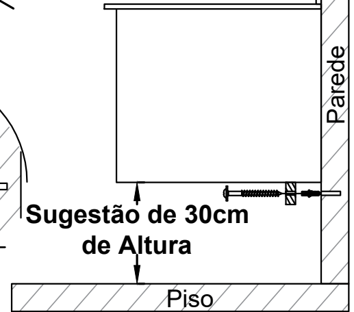
Detalhe C
