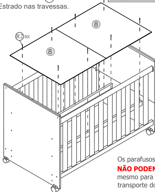
Figura 1 - Fixação do Estrado nas travessas.
